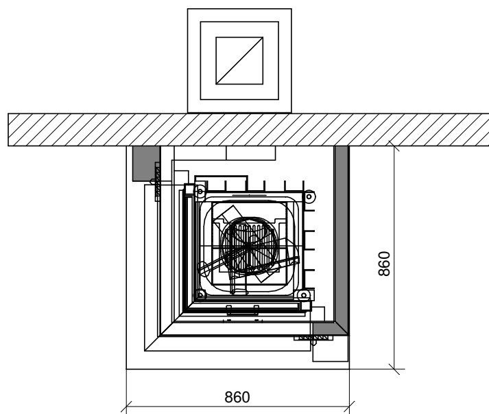
Draufsicht
