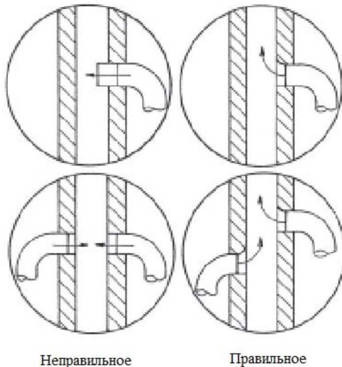
Рис. 1. ПОДСОЕДИНЕНИЕ К ТРУБЕ (ДЫМОХОДУ)
